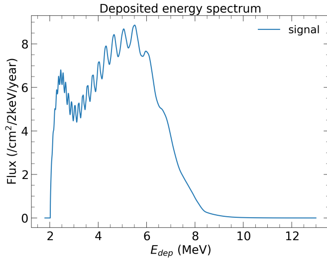
图 4-4 沉积能量能谱
