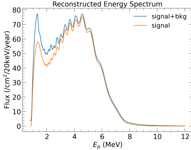
图 4-5 重建能量能谱
