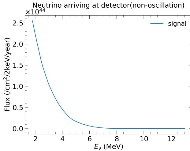
图 4-1 修正后的反中微子能谱 \phi'_r(E_\nu, t)
