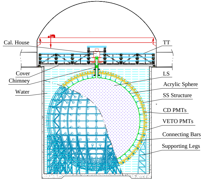
图 1-2 JUNO 的探测器示意图 [1] 。
