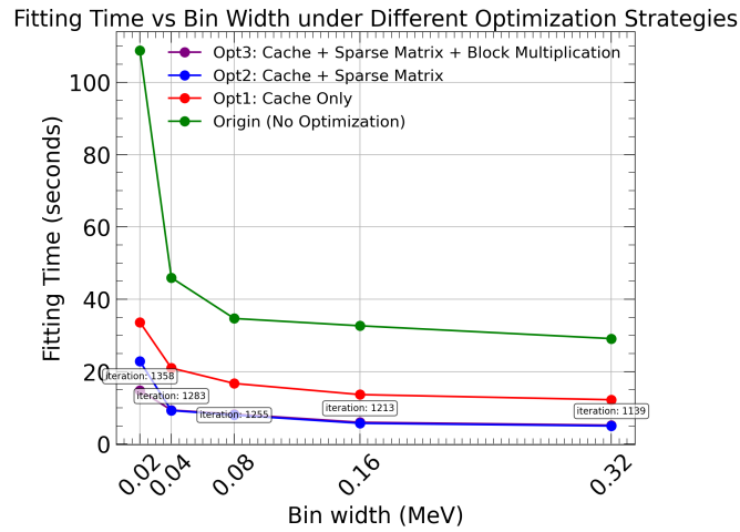
图 3-7 单次完整拟合耗时随重建能量能谱 bin 宽的变化。横轴为重建能量能谱直方图的 bin 宽 (MeV)；纵轴为单次完整拟合的时间 (秒)。曲线对应不同的优化配置：绿色—基线 (无优化)；红色—仅缓存；蓝色—缓存 + 稀疏 (CSR) 存储；品红色—缓存 + 稀疏 + 分块 (tiled) 乘法。每个点均在相同的能量区间 [0.8, 12.0] MeV 下通过不同等距箱数计算得到。
