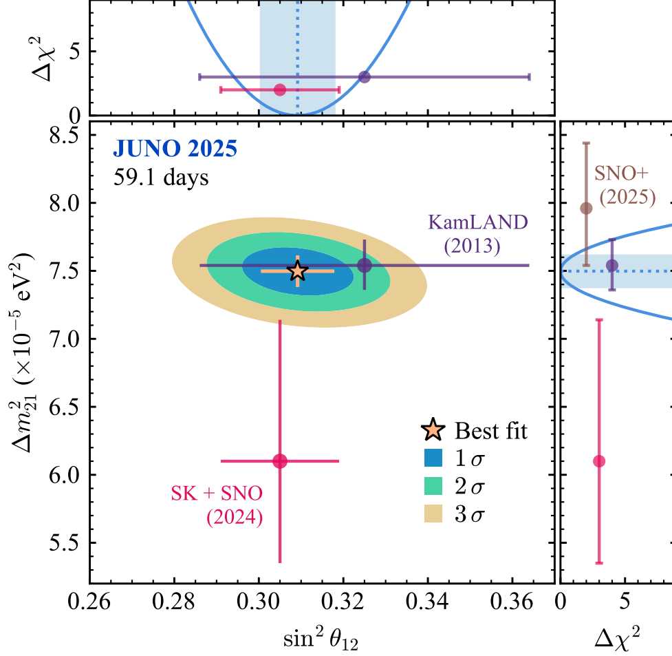
图 1-4 基于 2025 年 59.1 天 JUNO 数据，通过对反应堆反中微子提示能谱进行谱拟合得到的太阳振荡参数 \sin^2 \theta_{12} 与 \Delta m_{21}^2 的约束结果。阴影椭圆区域分别对应 1\sigma 、 2\sigma 和 3\sigma 置信区间。上方（右侧）面板给出了对另一参数进行 profile 处理后得到的 \sin^2 \theta_{12} ( \Delta m_{21}^2 ) 的一维 \Delta\chi^2 分布。星号表示 JUNO 的最佳拟合值，误差棒表示对应的一维 1\sigma 置信区间。同时给出了 KamLAND (2013)、SNO+ (2025) 以及 Super-Kamiokande 与 SNO 联合分析 (2024) 的结果以作比较。
