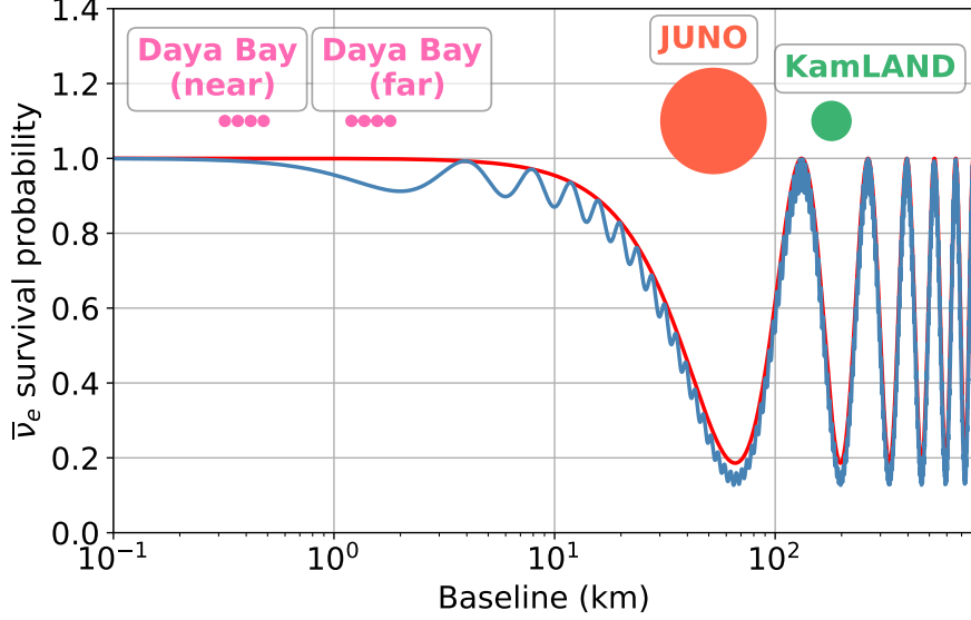
图 1-1 反应堆反中微子在不同基线下的存活概率。红曲线为由 \Delta m_{21}^2 驱动的慢振荡（太阳项），蓝曲线为包含由 \Delta m_{3e}^2 驱动的快振荡在内的三味总存活概率。图中标示了 JUNO（橙色，基线约 52.5 km，接近太阳振荡极大值）、大亚湾（粉色，近/远基线）和 KamLAND（绿色）的实验基线位置；图片来自文献 [20]
