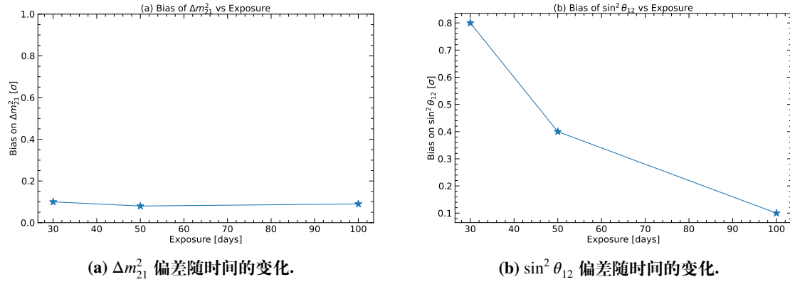
图 4-1 太阳振荡参数偏差随曝光时间的演化。(a) \Delta m^2_{21} 的偏差；(b) \sin^2 \theta_{12} 的偏差。
