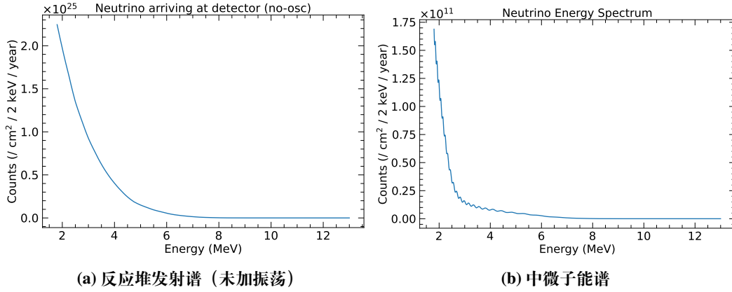
图 2-4 (a) 反应堆发射谱 (未加振荡): 按裂变同位素加权并经归一化的电子反中微子能量分布; (b) 加入振荡与几何衰减后的探测器处预期能谱: 将发射谱与存活概率以及 1/4\pi L^2 因子相乘并按能量分 bin 得到的结果 (单位为每 cm 2 每年每能量 bin 计数)。
