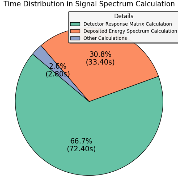
图 3-3 能谱计算内部的时间构成。探测器响应矩阵的计算（绿色）占多数，其次是沉积能量谱的生成（橙色），其余任务占比很小（蓝色）。
