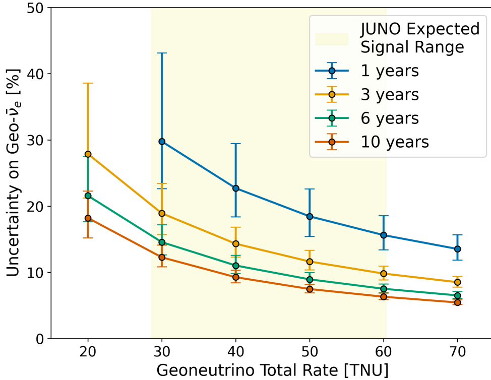
图 1-8 JUNO 对地球中微子总信号的预期测量精度。图中给出了在假设 \text{Th}/\text{U} 比为球粒陨石比例条件下，JUNO 对地球中微子总信号（单位：TNU）的预期相对不确定度随总信号强度变化关系。蓝色、橙色、绿色和红色曲线分别对应 1 年、3 年、6 年和 10 年运行时间的灵敏度预期。纵轴表示对地球中微子总信号的相对不确定度（%），横轴为地球中微子总事例率。黄色阴影区域表示不同 BSE（Bulk Silicate Earth）模型及岩石圈贡献预测所给出的 1\sigma 信号区间。结果表明，随着运行时间增加，统计不确定度显著降低，在 10 年运行条件下可实现约 5%–7% 量级的测量精度，从而对地球内部放射性元素分布模型形成重要约束。图片来自文献 [30]
