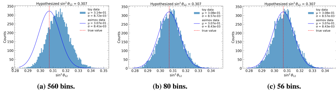
图 4-2 在 30 天曝光条件下，不同重建能谱分 bin 数目下 \sin^2 \theta_{12} 最佳拟合值在 10,000 个伪实验中的分布。
