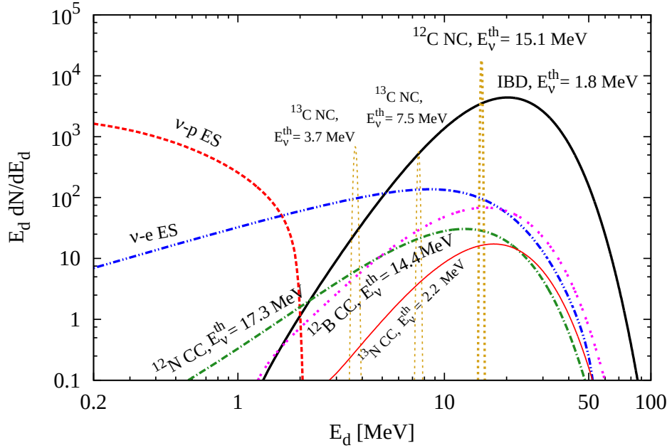
图 1-7 JUNO 探测器中不同超新星中微子相互作用通道的沉积能量分布。图中给出了在一次典型银河系核心坍缩超新星爆发条件下，JUNO 探测器内不同反应通道的可观沉积能量 E_d 分布，包括反 \beta 衰变 (IBD, \bar{\nu}_e + p \rightarrow e^+ + n )、电子弹性散射 ( \nu -e ES)、质子弹性散射 ( \nu -p ES)、以及在 ^{12}\text{C} 和 ^{13}\text{C} 上的带电流 (CC) 与中性流 (NC) 反应。图中同时标注了各反应的能量阈值 E_v^{\text{th}} 。可以看到，IBD 通道在数十 MeV 能区贡献最大，是 JUNO 探测超新星 \bar{\nu}_e 的主导通道；图片来自文献 [1]
