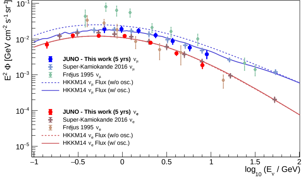
图 1-5 JUNO 对大气中微子能谱的灵敏度预期与现有实验结果比较。图中给出了在 5 年运行时间下，JUNO 对大气中微子通量 E^2\Phi 的预期测量结果（蓝色为 \nu_\mu ，红色为 \nu_e ），并与 Super-Kamiokande 2016 年测量结果以及 Fréjus 1995 年数据进行比较。同时给出了 Honda-Kajita-Kasahara-Midorikawa (HKKM14) 大气中微子通量模型在考虑振荡（实线）和不考虑振荡（虚线）情况下的理论预期。横轴为中微子能量的对数刻度 \log_{10}(E_\nu/\text{GeV}) ，纵轴为 E^2\Phi 。可以看出，在 GeV 能区，振荡效应对 \nu_\mu 通量产生显著压低，而 \nu_e 通量则表现出相对增强或形状变化。JUNO 的测量精度在多 GeV 区间内具有良好的统计灵敏度，可用于检验大气中微子振荡模型并辅助质量顺序分析。该图来自文献 [1]
