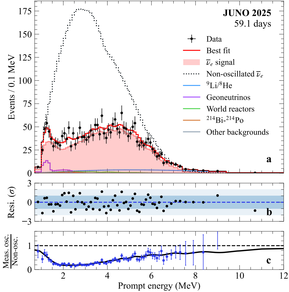
图 1-3 (a) 黑点为经过事例挑选后的 IBD 候选事例的测量值 (带统计误差), 红色实线为包含振荡效应的最佳拟合模型, 红色阴影区为拟合出的反中微子信号分量。黑色虚线为若无振荡时的反应堆中微子预期谱。其他有色实线分别表示主要本底成分 (例如宇宙线次级粒子 {}^9\text{Li}/{}^8\text{He} 、地球中微子、来自全球反应堆的中微子贡献、 {}^{214}\text{Bi}-{}^{214}\text{Po} 等)。(b) 数据与完整模型之间的残差及其一致性检验。(c) 测得的振荡后谱与无振荡预测之比, 显示能谱上的振荡形状特征。该图直接展示了在短期运行下 JUNO 对 IBD 能谱的重建能力与振荡信号的显著性 (见文献 [20] )。
