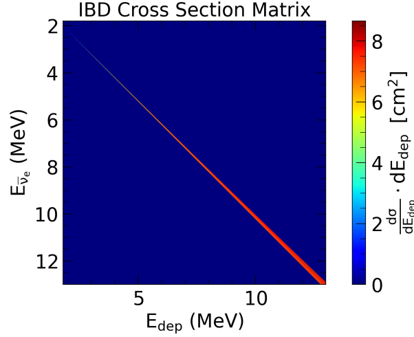
图 4-4 IBD 微分散射截面矩阵 \frac{d\sigma}{dE_{\text{dep}}}(E_{\text{dep}}, E_{\bar{\nu}_e}) 的热力图（色标单位为 10^{-44} \text{ cm}^2 / 2 \text{ keV} ）。横轴为沉积能量 E_{\text{dep}} (MeV)，纵轴为入射反中微子能量 E_{\bar{\nu}_e} (MeV)；颜色越暖表示差分截面值越大。图中清晰可见主对角带，表明矩阵适合采用带状稀疏表示以加速谱的构造与拟合。
