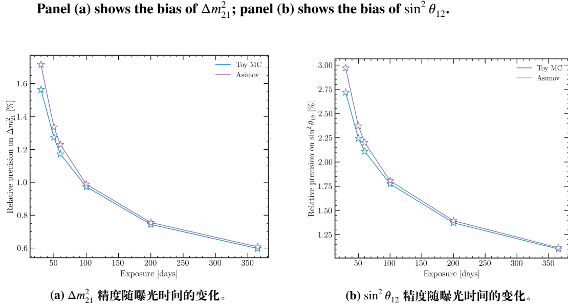
图 5-2 太阳振荡参数精度随曝光时间的演化。(a) \Delta m_{21}^2 的精度；(b) \sin^2 \theta_{12} 的精度。
