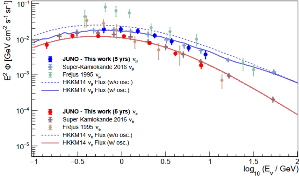
图 1-1 JUNO 对大气中微子能谱的灵敏度预期与现有实验结果比较。图中给出了在 5 年运行时间下，JUNO 对大气中微子通量 E^2\Phi 的预期测量结果（蓝色为 \nu_\mu ，红色为 \nu_e ），并与 Super-Kamiokande 2016 年测量结果以及 Fréjus 1995 年数据进行比较。同时给出了 Honda-Kajita-Kasahara-Midorikawa (HKKM14) 大气中微子通量模型在考虑振荡（实线）和不考虑振荡（虚线）情况下的理论预期。横轴为中微子能量的对数刻度 \log_{10}(E_\nu/\text{GeV}) ，纵轴为 E^2\Phi 。可以看出，在 GeV 能区，振荡效应对 \nu_\mu 通量产生显著压低，而 \nu_e 通量则表现出相对增强或形状变化。JUNO 的测量精度在多 GeV 区间内具有良好的统计灵敏度，可用于检验大气中微子振荡模型并辅助质量顺序分析。该图来自文献 [7]
