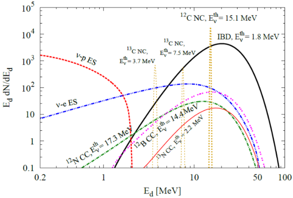
图 1-3 JUNO 探测器中不同超新星中微子相互作用通道的沉积能量分布。图中给出了在一次典型银河系核心坍缩超新星爆发条件下，JUNO 探测器内不同反应通道的可观沉积能量 E_d 分布，包括反 \beta 衰变 (IBD, \bar{\nu}_e + p \rightarrow e^+ + n )、电子弹性散射 ( \nu -e ES)、质子弹性散射 ( \nu -p ES)、以及在 ^{12}\text{C} 和 ^{13}\text{C} 上的带电流 (CC) 与中性流 (NC) 反应。图中同时标注了各反应的能量阈值 E_\nu^{\text{th}} 。可以看到，IBD 通道在数十 MeV 能区贡献最大，是 JUNO 探测超新星 \bar{\nu}_e 的主导通道；
