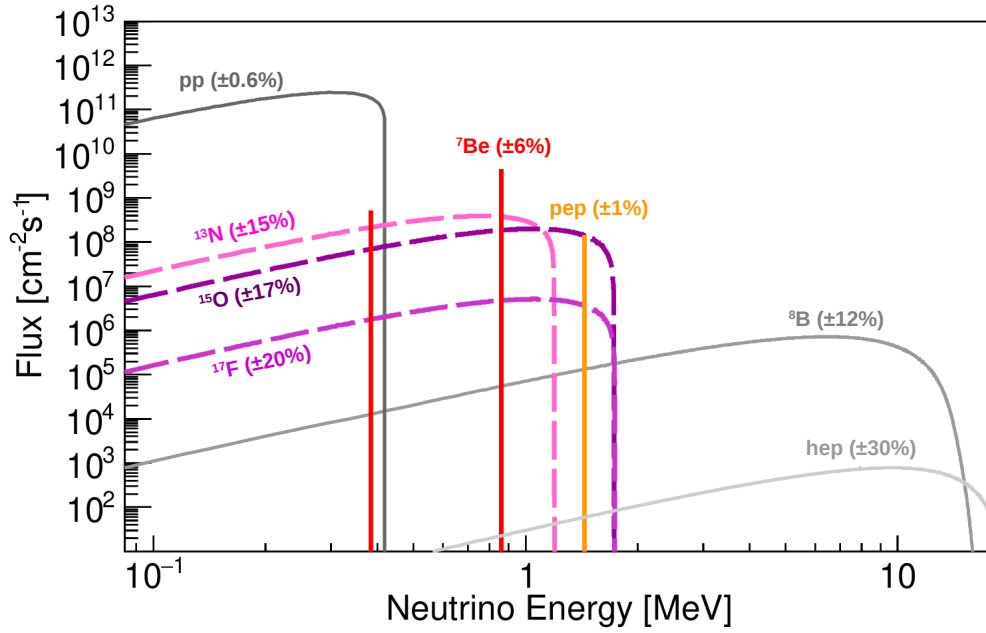
图 1-2 太阳中微子能谱及理论通量预测。图中给出了标准太阳模型 (Standard Solar Model, SSM) 预测的各类太阳中微子通量随能量变化关系, 包括 pp、 {}^7\text{Be} 、pep、 {}^8\text{B} 、hep 以及 CNO 循环产生的 {}^{13}\text{N} 、 {}^{15}\text{O} 、 {}^{17}\text{F} 中微子。不同曲线对应不同反应来源, 括号中标注为理论通量的不确定度。红色和橙色竖线分别标示了 JUNO 对 {}^7\text{Be} 和 pep 单能谱太阳中微子的主要灵敏能区。该图展示了低能 pp 与 {}^7\text{Be} 中微子在太阳中微子总通量中的主导地位, 以及高能 {}^8\text{B} 与 hep 中微子在高能区的重要贡献。图片来自文献 [8]
