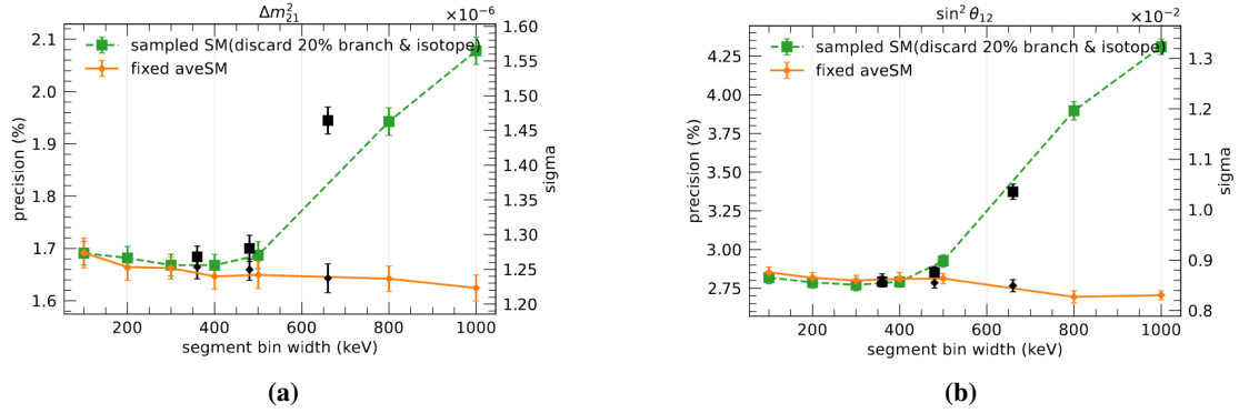
图 5-3 (a) \Delta m^2_{21} 与 (b) \sin^2 \theta_{12} 的测量精度随反应堆谱段宽的变化关系。绿色标记 / 曲线表示在对 Summation 模型进行扰动（随机丢弃 20% 的裂变分支 / 同位素）时得到的结果；橙色标记 / 曲线为固定平均 Summation 模型下的基线精度。黑色点对应以探测器能量分辨为驱动的分段（energy-resolution-driven segmentation），彩色曲线点对应对反应堆谱做的均匀分段。误差线表示由重复 toys/fits 给出的统计不确定度。在约 300 keV 附近，额外的模型相关系统不确定度达到最小，表明在模型灵活性与可用统计约束之间达到了较优折中。
