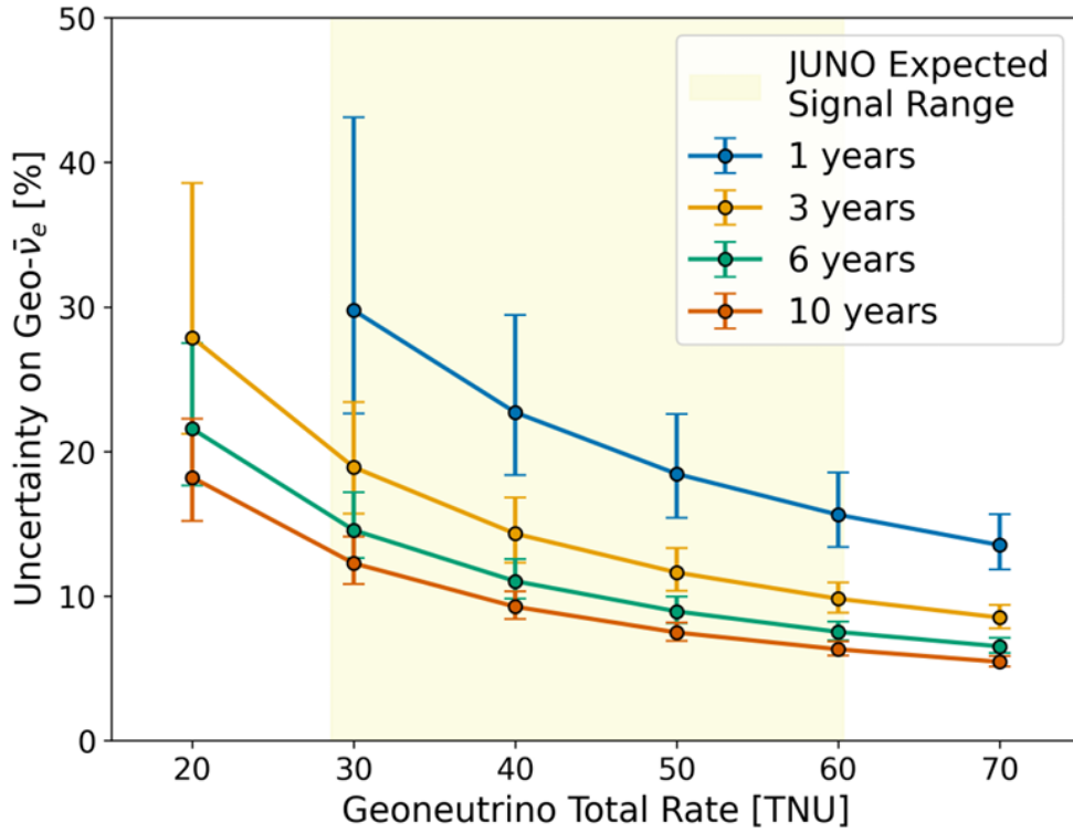
图 1-4 JUNO 对地球中微子总信号的预期测量精度。图中给出了在假设 Th/U 比为球粒陨石比例条件下，JUNO 对地球中微子总信号（单位：TNU）的预期相对不确定度随总信号强度变化关系。蓝色、橙色、绿色和红色曲线分别对应 1 年、3 年、6 年和 10 年运行时间的灵敏度预期。纵轴表示对地球中微子总信号的相对不确定度（%），横轴为地球中微子总事例率。黄色阴影区域表示不同 BSE（Bulk Silicate Earth）模型及岩石圈贡献预测所给出的 1\sigma 信号区间。结果表明，随着运行时间增加，统计不确定度显著降低，在 10 年运行条件下可实现约 5%–7% 量级的测量精度，从而对地球内部放射性元素分布模型形成重要约束。
