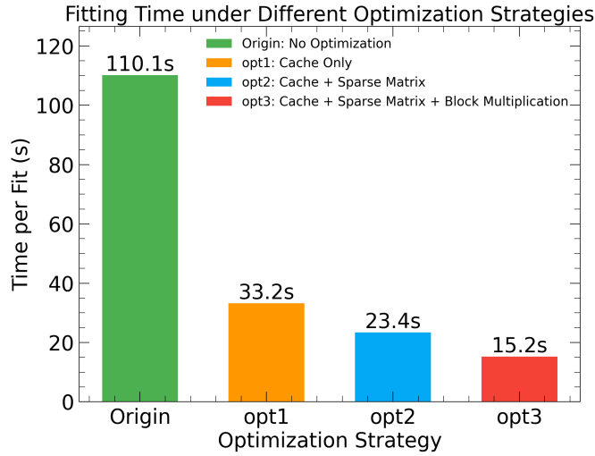
图 5-5 不同优化策略下单次拟合平均耗时比较。横坐标依次为：未经优化的基线实现 ( Origin )、仅启用缓存 ( opt1 )、缓存 + 差分截面稀疏表示 ( opt2 )、缓存 + 稀疏表示 + 分块乘法 ( opt3 )。纵坐标为单次拟合的平均耗时时间 (秒)。柱状图展示了随着逐步应用优化策略, 运行时间的逐级下降; 其中 opt3 达到最短的拟合时间。
