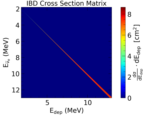
图 5-4 IBD 微分散射截面矩阵 \frac{d\sigma}{dE_{\text{dep}}}(E_{\text{dep}}, E_{\bar{\nu}}) 的热力图（色标单位为 10^{-44} \text{ cm}^2 / 2 \text{ keV} ）。横轴为沉积能量 E_{\text{dep}} (MeV)，纵轴为入射反中微子能量 E_{\bar{\nu}} (MeV)；颜色越暖表示差分截面值越大。图中清晰可见主对角带，表明矩阵适合采用带状稀疏表示以加速谱的构造与拟合。
