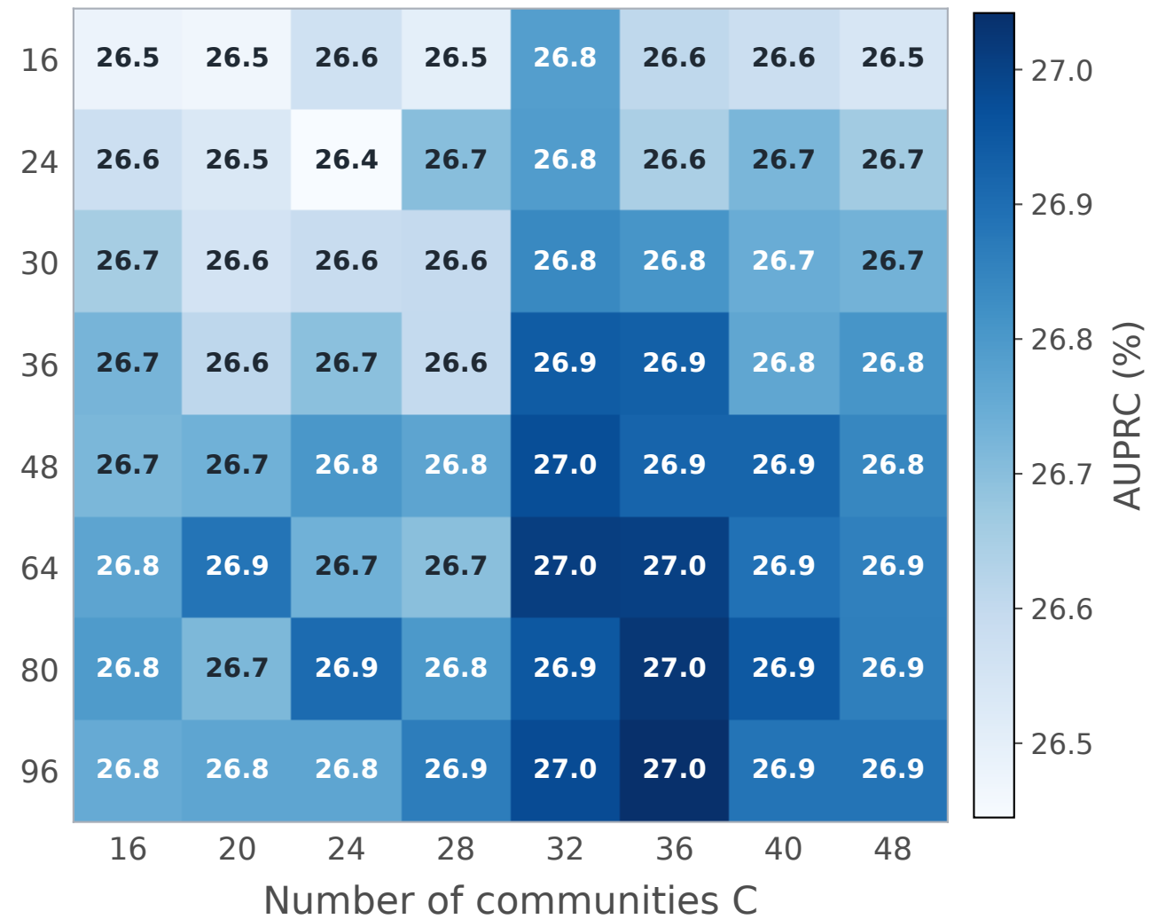
(b) AUPRC
