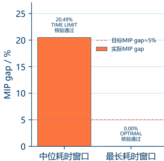
(a) 代表窗口MIP gap与独立核验结果
