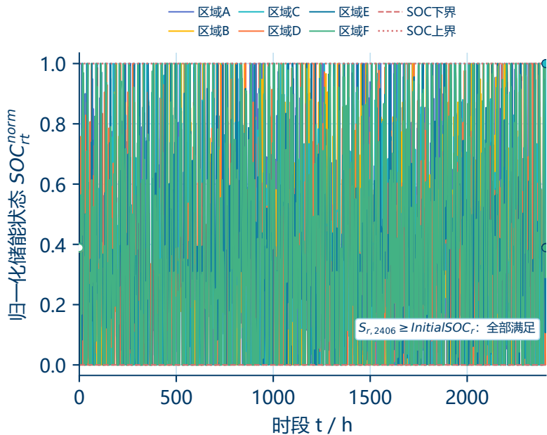
(b) 六区域SOC可行性与终端恢复
