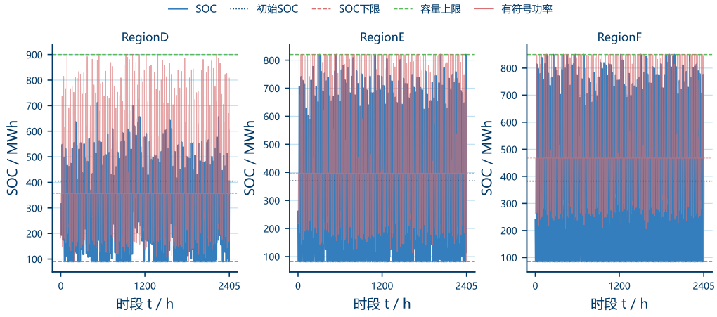
(b) RegionD-F SOC与充放电时序特征
