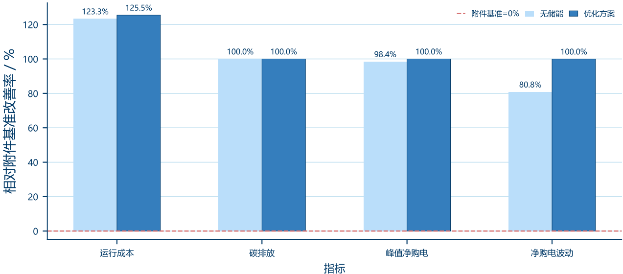
(a) 无储能与优化方案相对附件基准的四指标改善率
