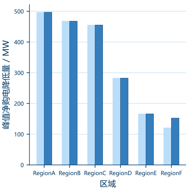
(b) 六区域峰值净购电改善
