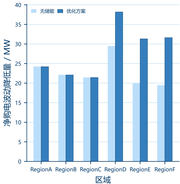
(c) 六区域净购电波动改善
