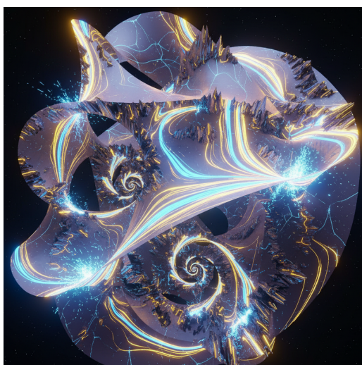
图 73.2: 复杂系统的几何结构上流动示意图
