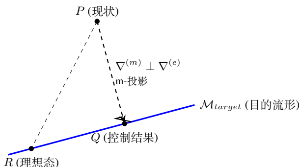
图 27.1: 广义勾股定理保证了宏观控制总是缩短与理想态的距离
