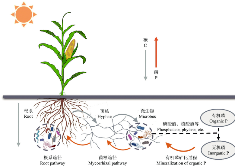
图 62.4: 菌丝网络中的物质交换与网络优化示意图
