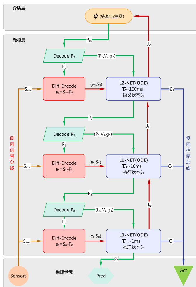
图 71.1: 微观层 ODE 网络架构示意图
