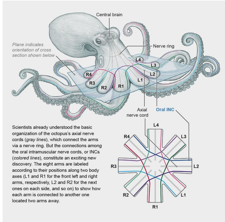
图 57.3: 章鱼的大脑结构示意图
