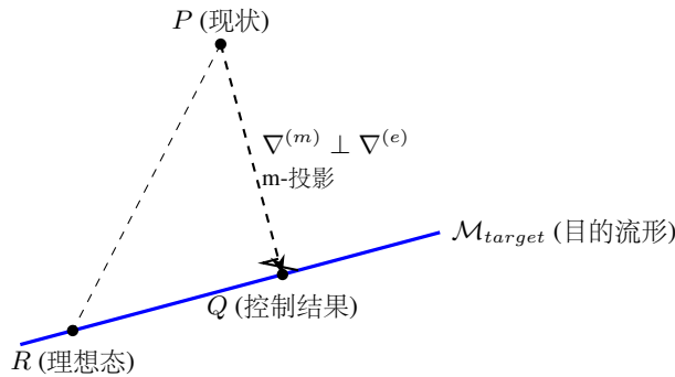
图 26.1: 广义勾股定理保证了宏观控制总是缩短与理想态的距离
