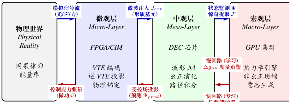
图 74.1: HSF-HD SoC 混合动力学流图 (水平全闭环)
