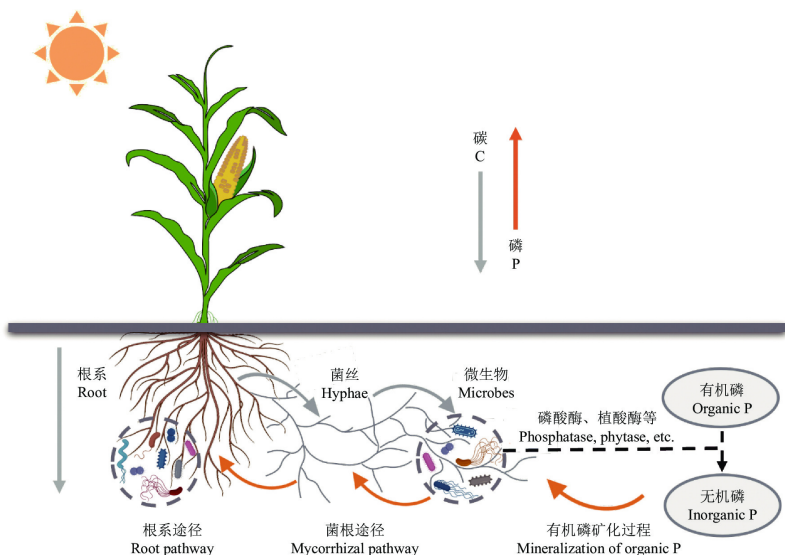
图 60.4: 菌丝网络中的物质交换与网络优化示意图
