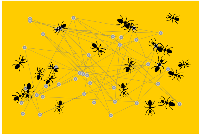
图 60.1: 蚁群中的信息素场示意图
