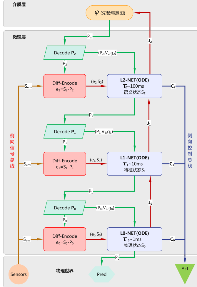
图 74.1: 微观层 ODE 网络架构示意图
