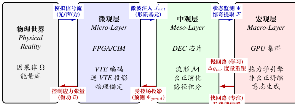
图 70.1: HSF-HD SoC 混合动力学流图 (水平全闭环)
