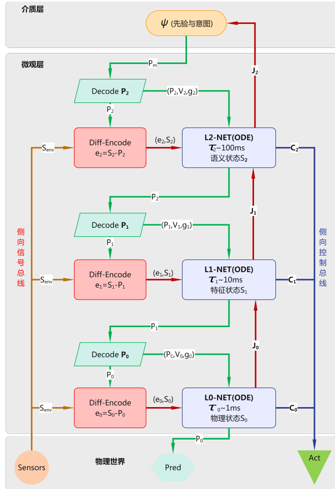
图 70.1: 微观层 ODE 网络架构示意图
