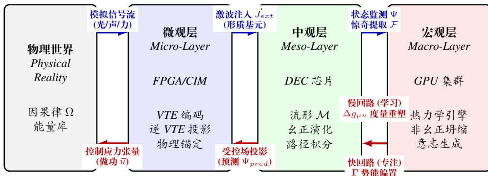
图 68.1: HSF-HD SoC 混合动力学流图 (水平全闭环)
