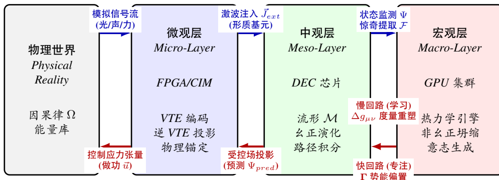
图 65.1: HSF-HD SoC 混合动力学流图 (水平全闭环)
