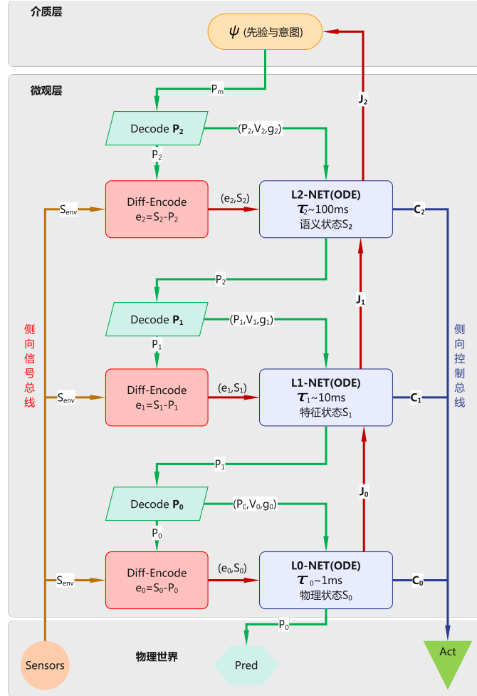
图 67.1: 微观层 ODE 网络架构示意图
