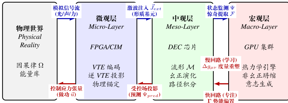
图 66.1: HSF-HD SoC 混合动力学流图 (水平全闭环)
