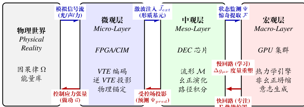
图 73.1: HSF-HD SoC 混合动力学流图 (水平全闭环)
