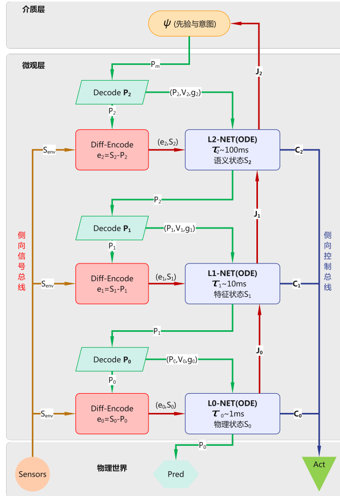
图 80.1: 微观层 ODE 网络架构示意图
