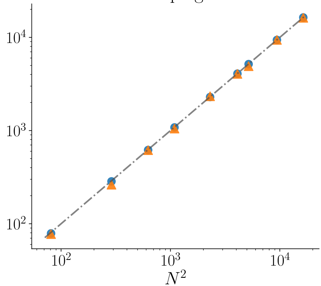
Doping
