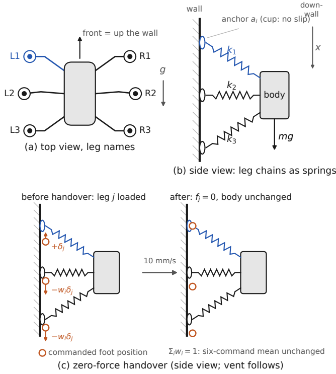
图 1. 平台与零力交接 (示意图)。(a) 俯视与腿命名: 机器人面朝墙的上方, 故 1 号腿为最上方一对。(b) 侧视: 每条吸附腿链相当于机体与足端锚点 a_i (不会打滑) 之间的一根弹簧 k_i ; 机体在自重 mg 下挂在这根弹簧上; x 沿墙向下计量。(c) 零力交接, 以一条上方腿 j 为例: 吸附中的脚都位于各自指令位置 (空心圆) 的上方, 即每条腿都被拉长。放气 j 之前, 其足端指令沿墙向上移动 \delta_j 直到弹簧松弛 ( f_j = 0 ), 各支撑足指令同时沿墙向下移动 w_j \delta_j , \sum_i w_i = 1 ; 机体的指令位置不变, 随后密封断开时已无可释放。[待办: 补 (d): 机器人在玻璃墙上的照片。]
