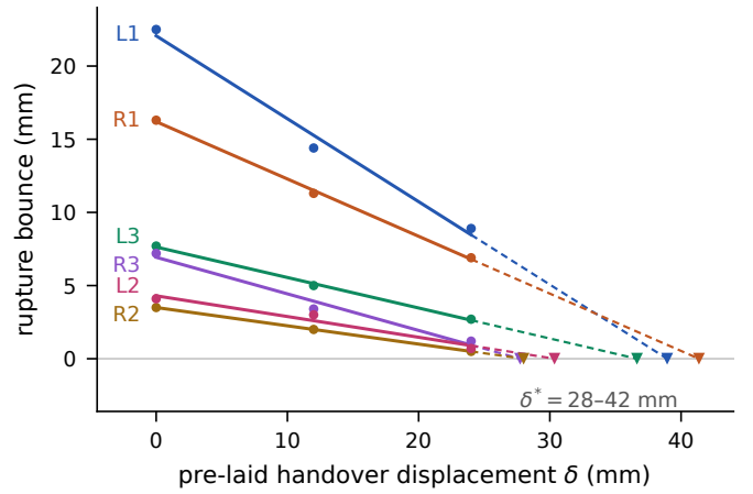
图 3. P1 验证: 破裂弹跳 vs. 放气前施加的卸载位移 \delta (三剂量标定第 2 轮, \delta = 0/12/24 \text{ mm} , 六腿同值)。六腿全部严格线性 (中点残差 \leq 1 \text{ mm} ); 斜率逐腿相差 4 倍 (刚度不均); 虚线外推至零弹跳给出标定目标 \delta_j^* = 28\text{--}42 \text{ mm} (三角)。
