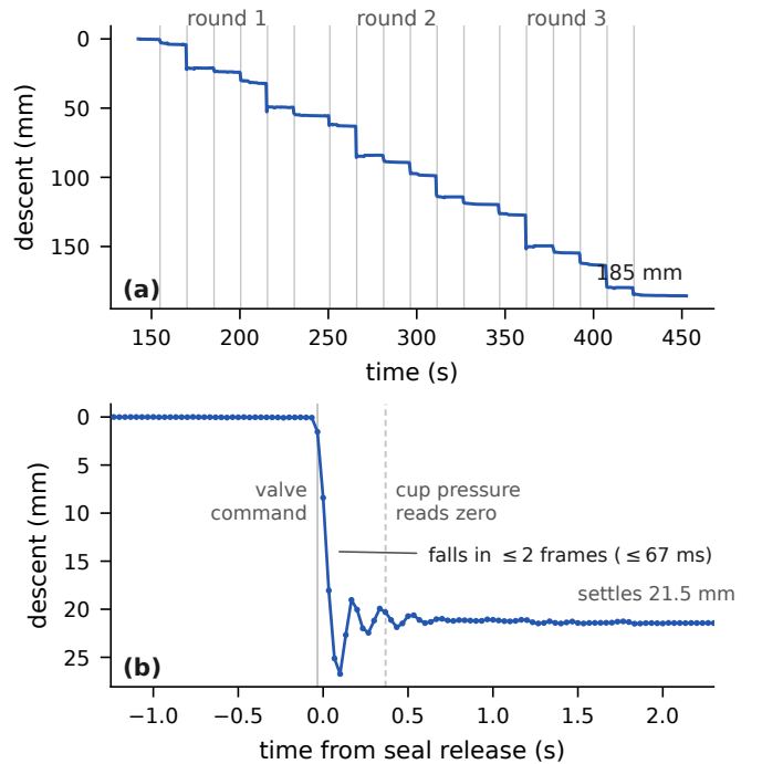
图 2. Vent-snap 棘轮 (基线, 重复 #1)。(a) 三轮原地踏步的机体沿墙位置: 185 mm 阶梯的每一级都与一次密封破裂 (灰色) 重合, 级间轨迹平坦。(b) 一次抬落 (L1, 第 2 轮) 的原始 30 fps 剖面, t=0 取追踪到的释放时刻: 释放前机体纹丝不动, 两帧内坠 21.5 mm 并带欠阻尼过冲 (峰 26.7 mm); 同一瞬间被释放的脚沿墙回弹 12.8 mm (图中未示)。日志的阅开指令与释放确认 (盘压归零) 两事件夹住机械释放; 两者相对视频的位位置带对时不确定度 (零点几秒)。
