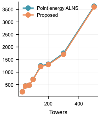
Makespan
