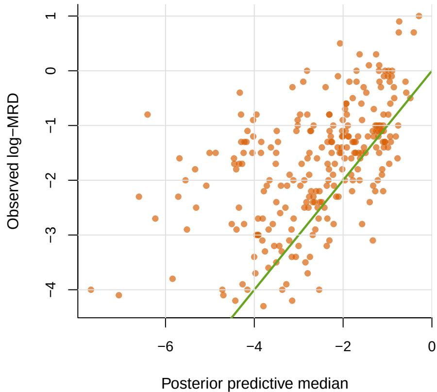
Posterior Predictive Check
