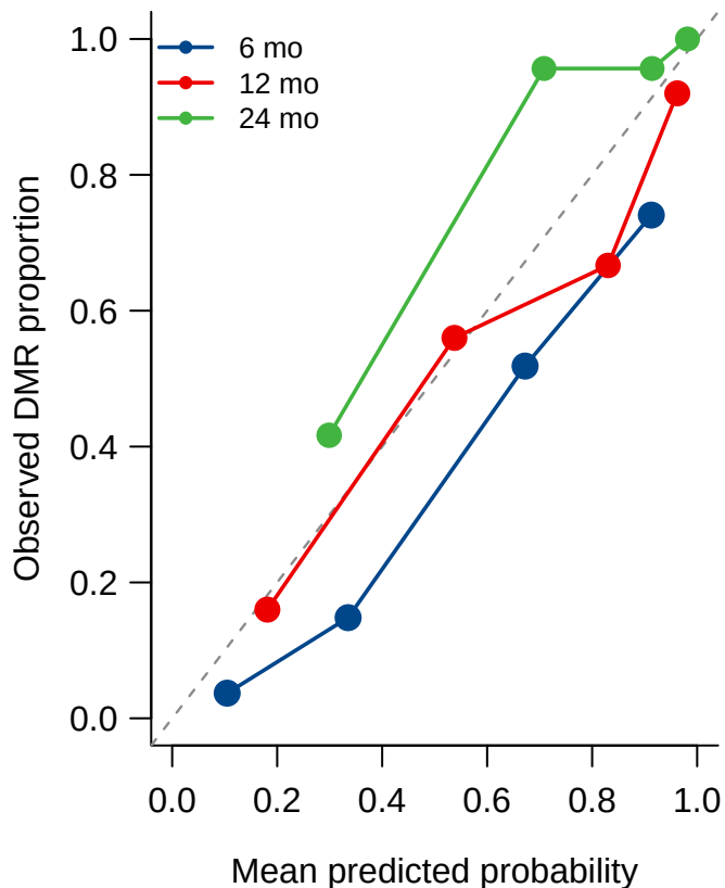
Original posterior
