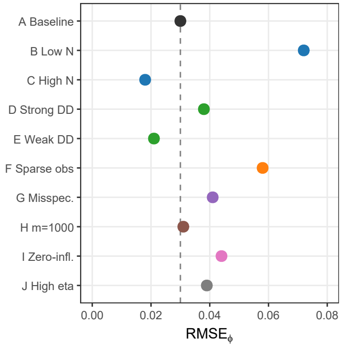
(a) Parameter recovery
