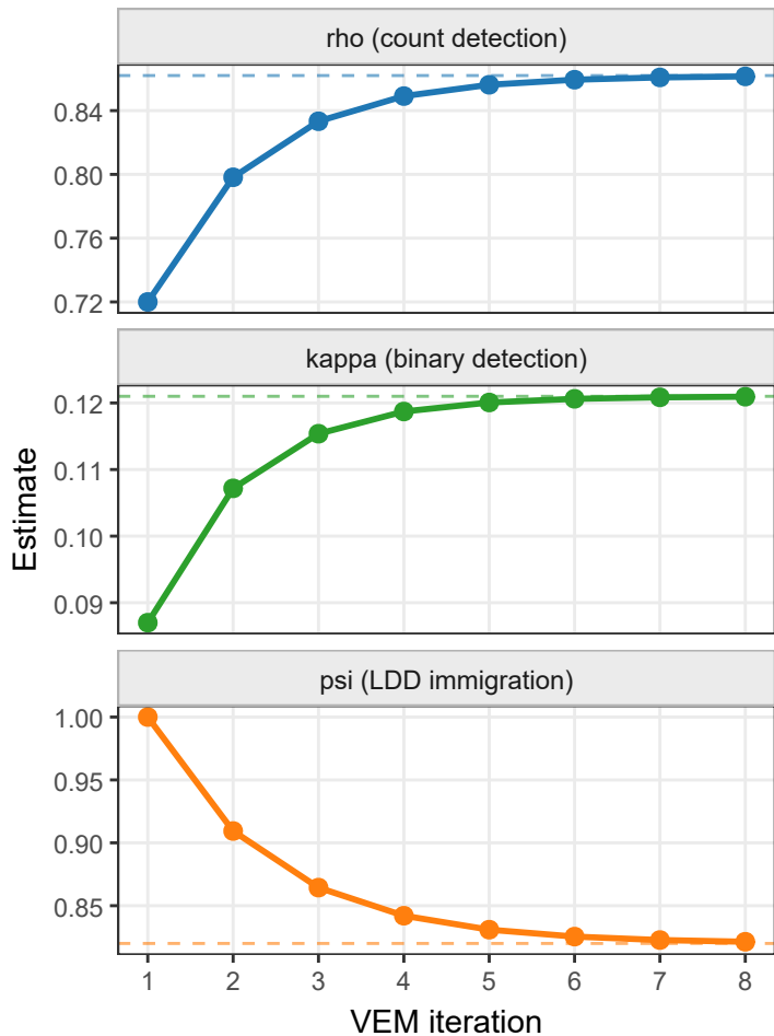
(a) Parameter convergence
