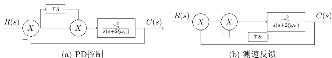
图 8: 二阶系统改善结构图
