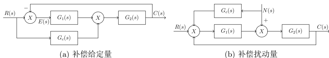
图 10: 前馈复合控制结构图
