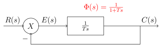
图 6: 一阶系统结构图
