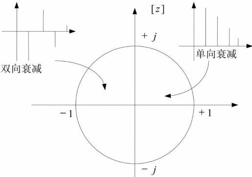
图 19: 动态响应
