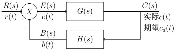
图 9: 稳态误差结构图
