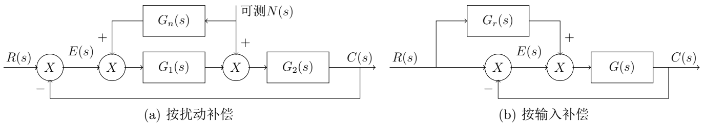
图 15: 复合校正结构图
