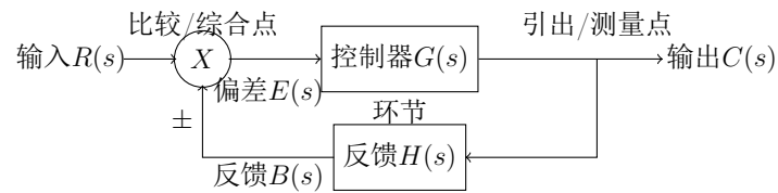
图 3: 结构图
