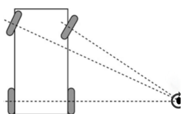
图 4: 瞬心
