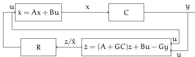
图 24: 龙伯格观测器结构图
