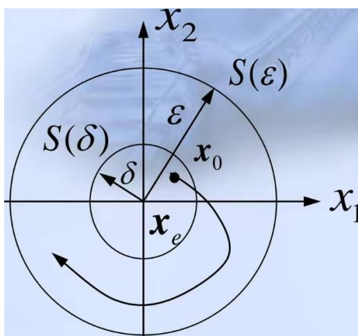
图 23: 轨迹示意图（李雅普诺夫意义下的稳定）
