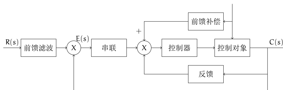
图 12: 校正结构图
