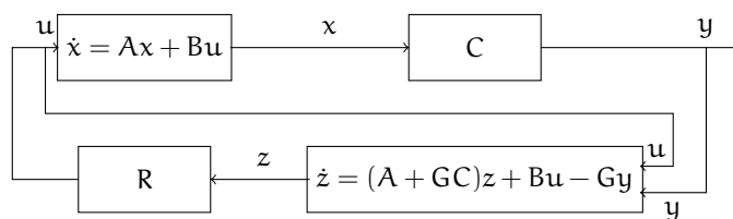
图 23: 龙伯格观测器结构图
