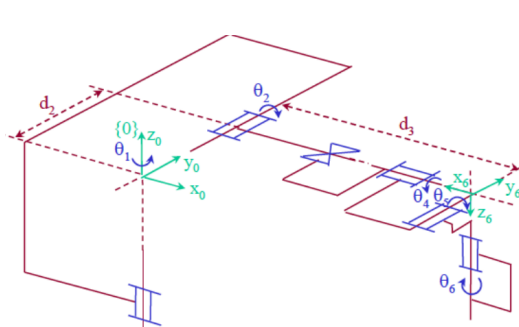
(a) 斯坦福臂结构图
