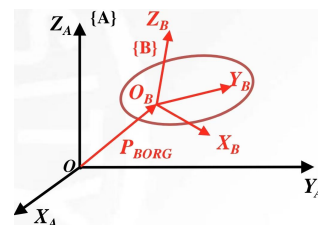
图 4: 刚体位姿
