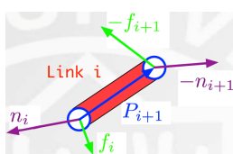
(a) 静力学受力分析
