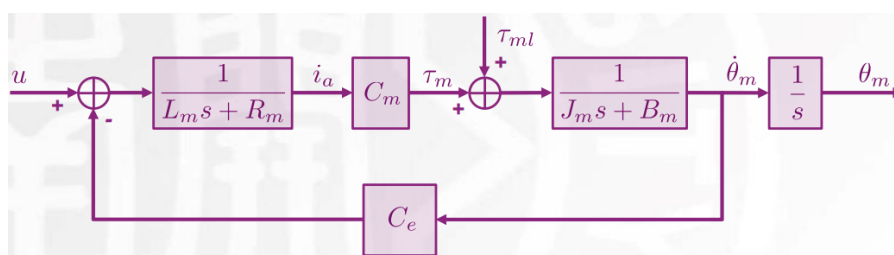
图 32: 电机动力学控制框图
