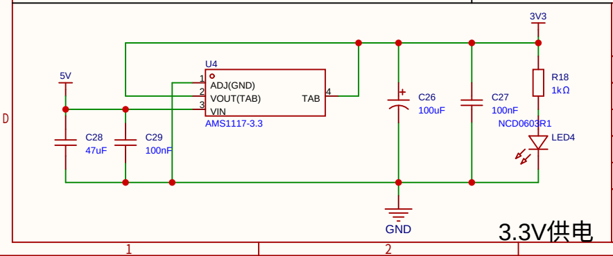
lora模组供电
