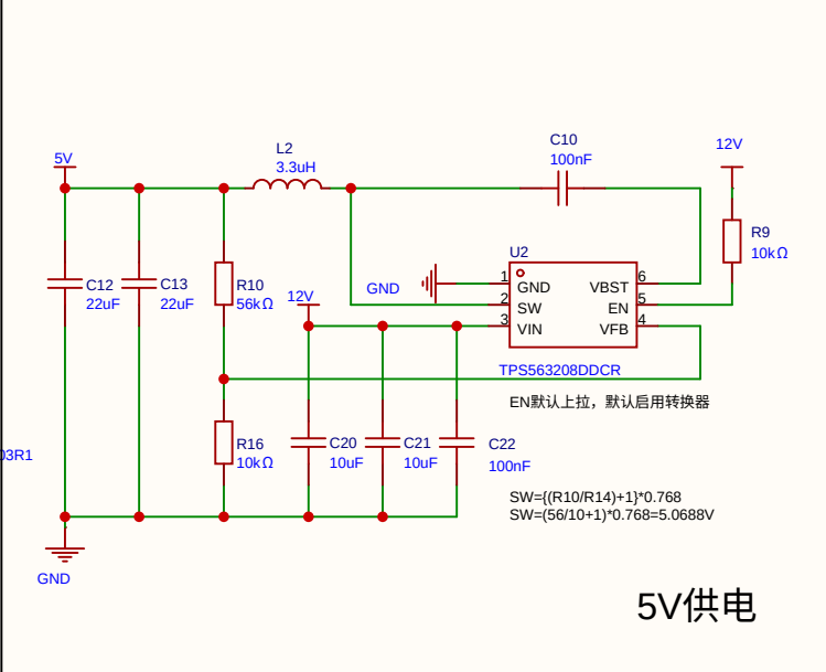
lora模组供电
