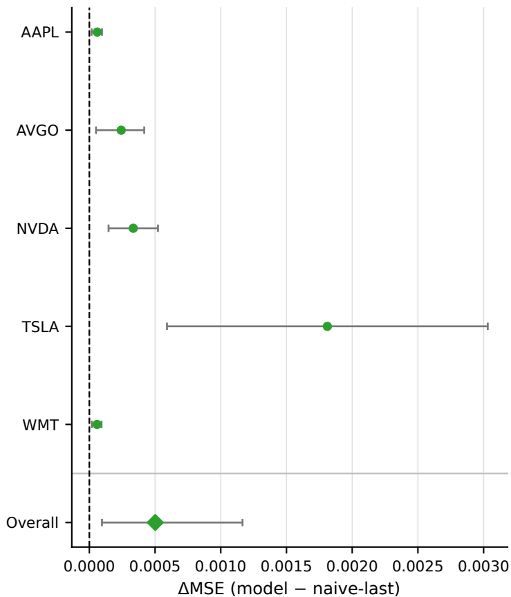
GRU
