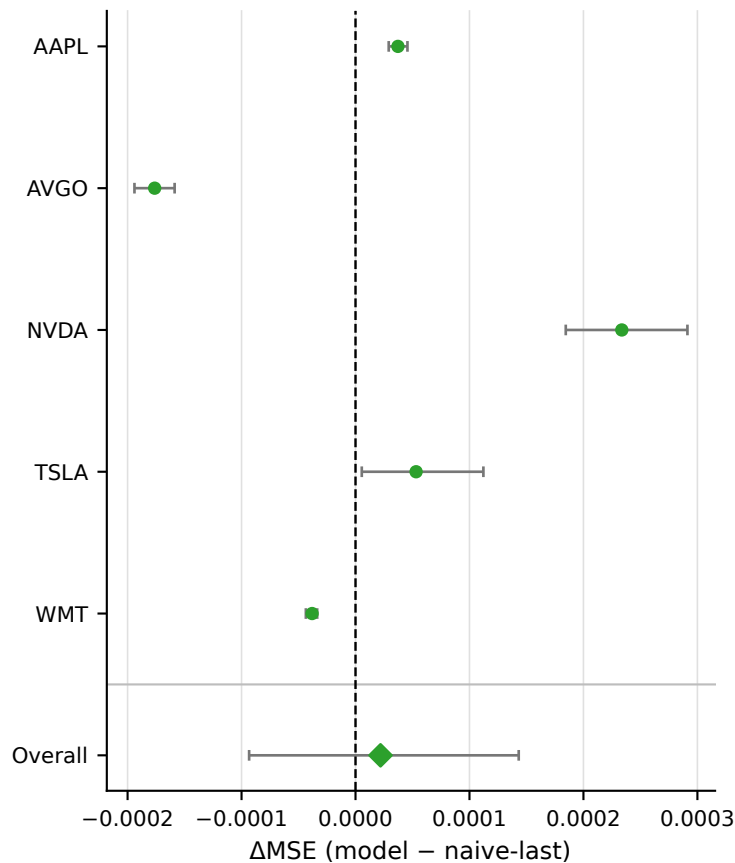
GRU
