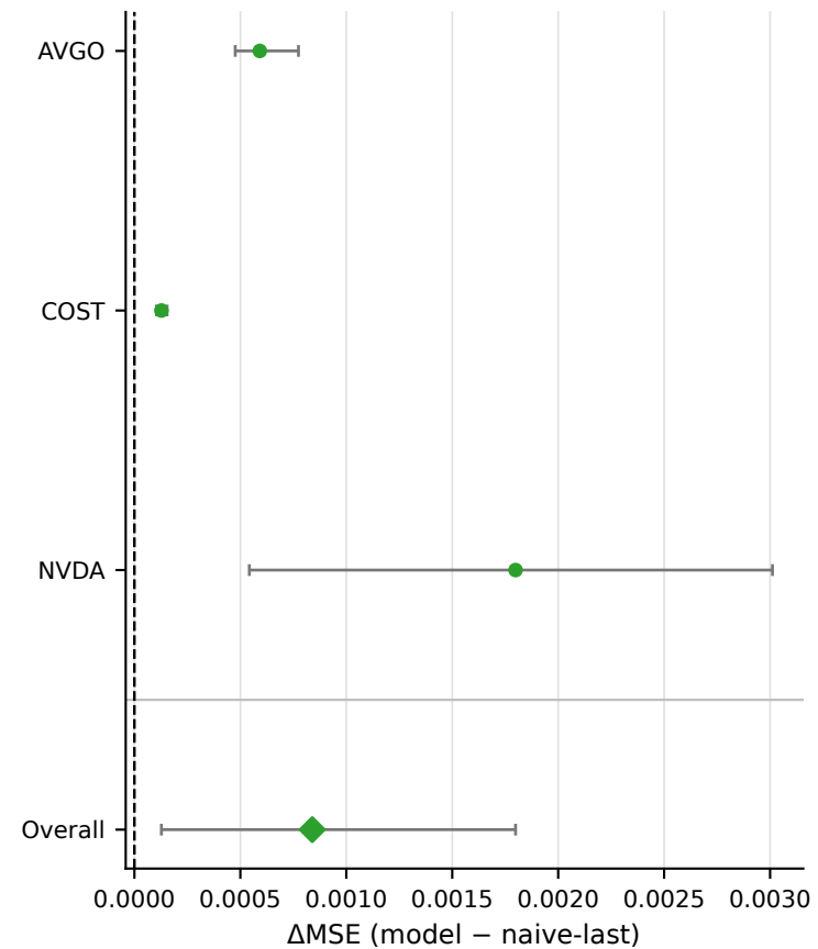
GRU
