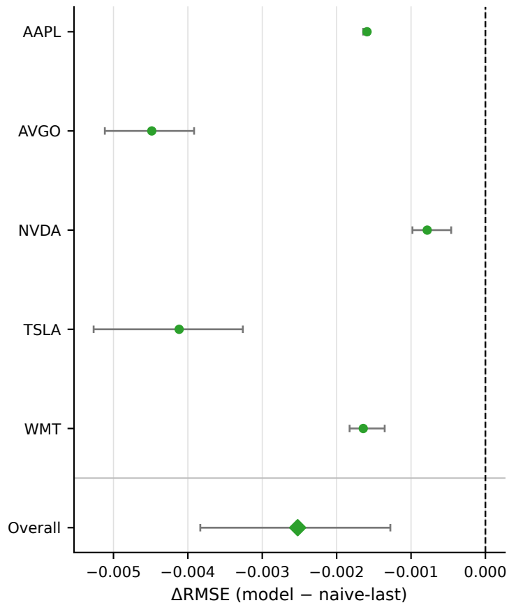
GRU
