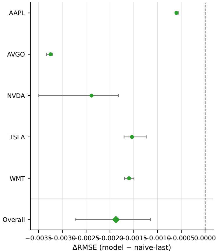
GRU
