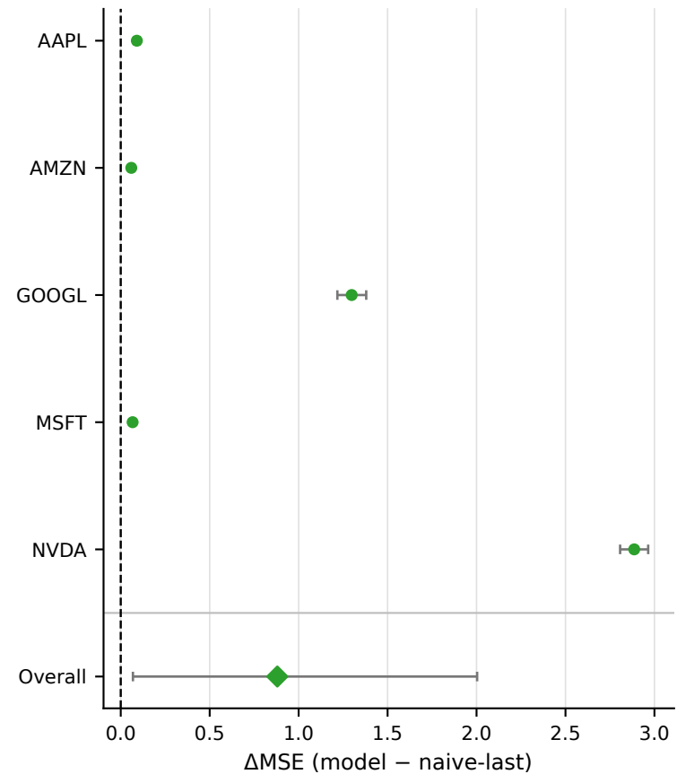
GRU
