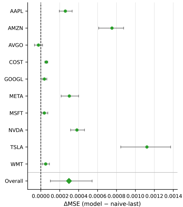
GRU
