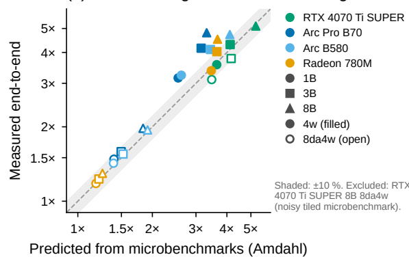
(d) Microkernel gains vs. model-level gains
