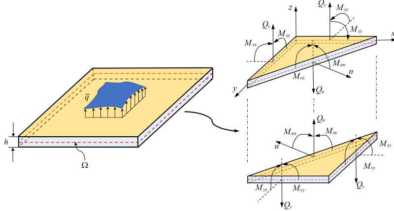
图 5.1 中厚板运动学及边界条件
