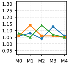
(b) RoPE
