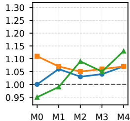
(d) Add
