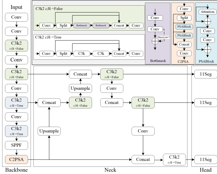
图 2-1 YOLO11s-Seg 主干与注意力结构示意图
