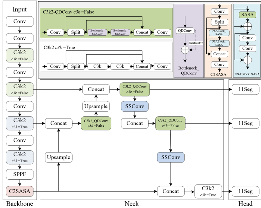
图 2-2 YOLO11-StackLite 整体结构
