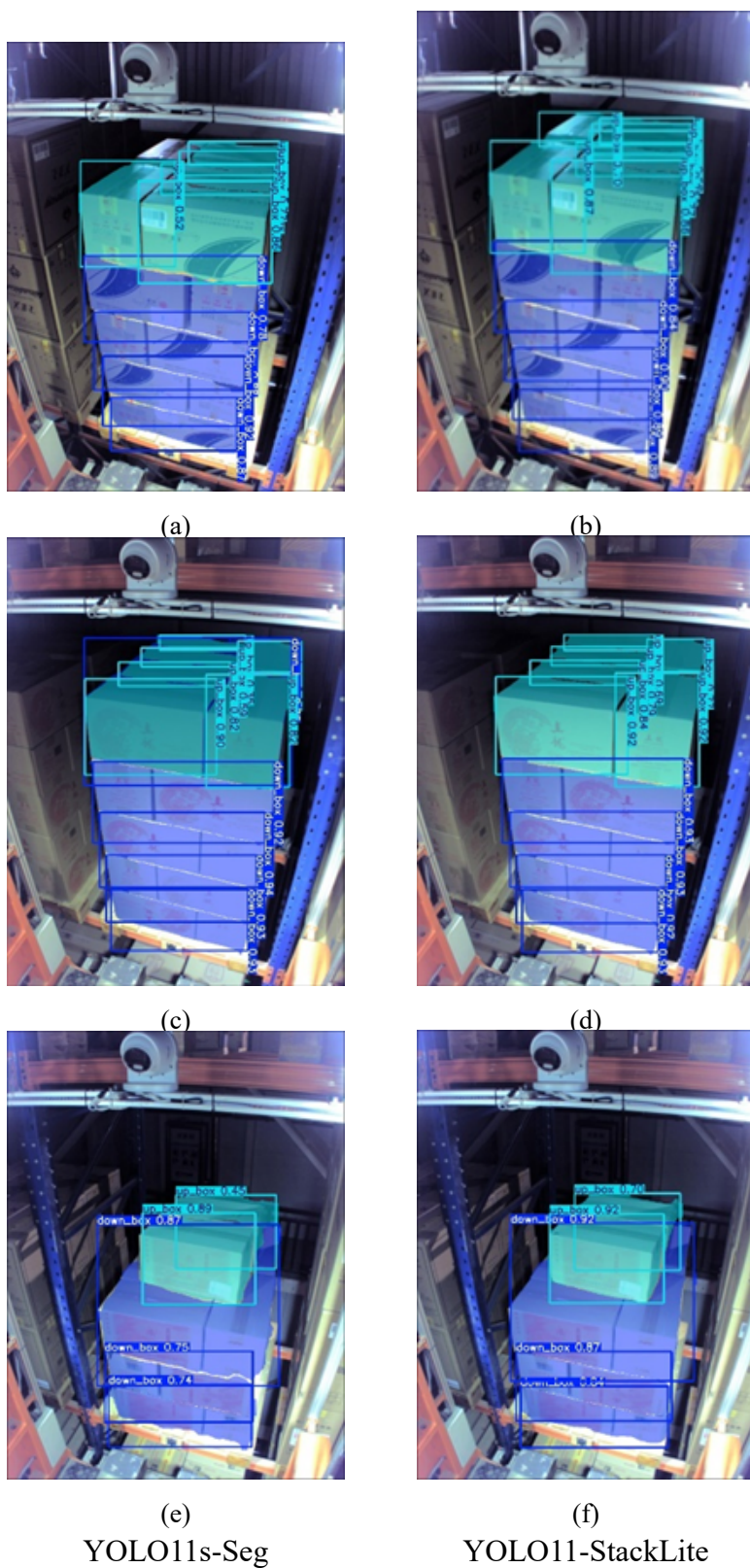
图 4-1 改进前后模型实例分割效果对比
