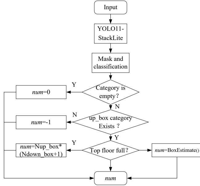
图 2-7 后处理数量估计流程示意图
