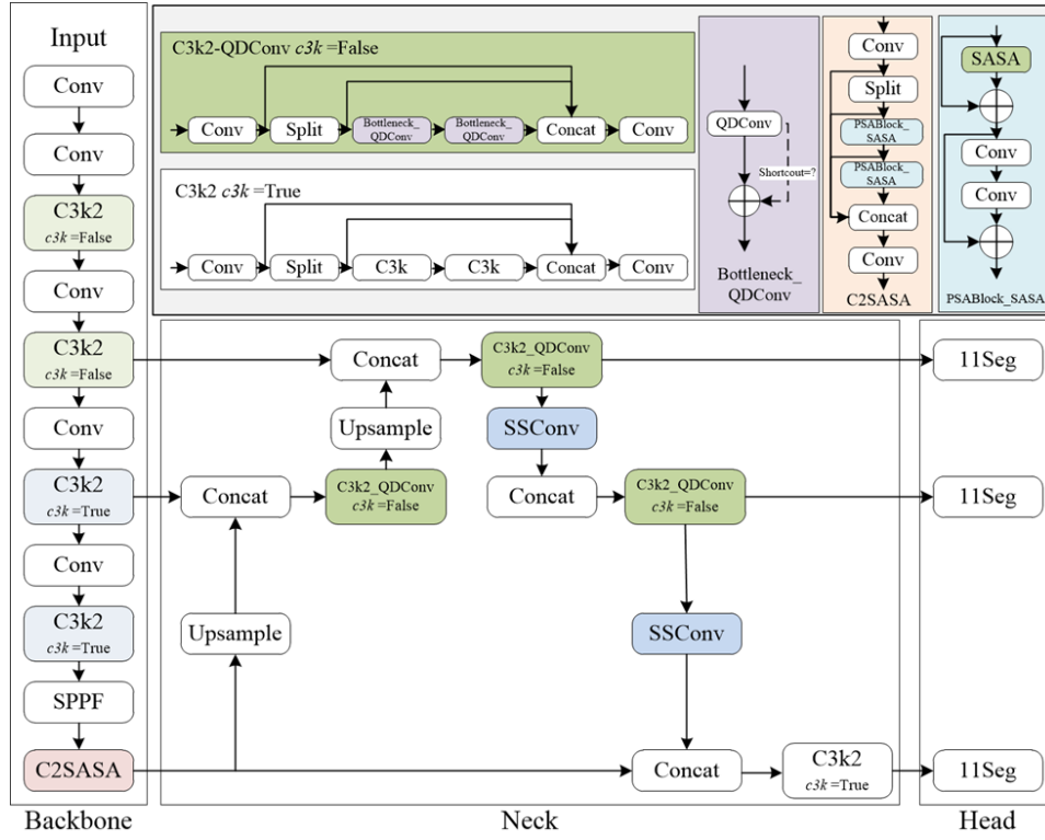
图 2-1 YOLO11s-Seg 主干与注意力结构示意图
