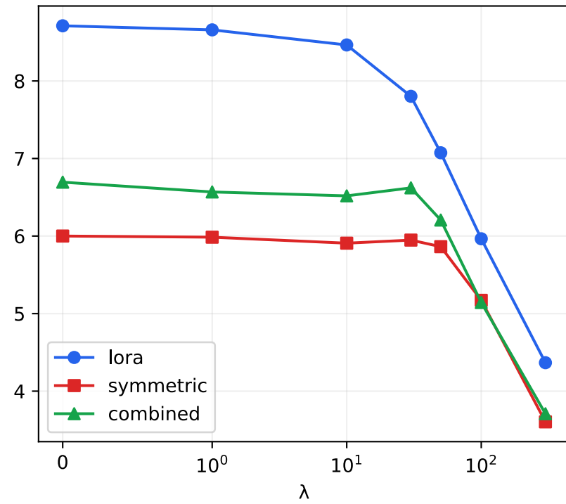
Parameter displacement A \rightarrow C
