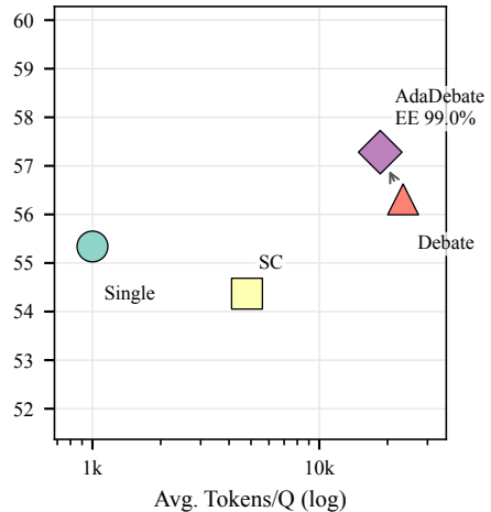
MultiRC (N=950)
